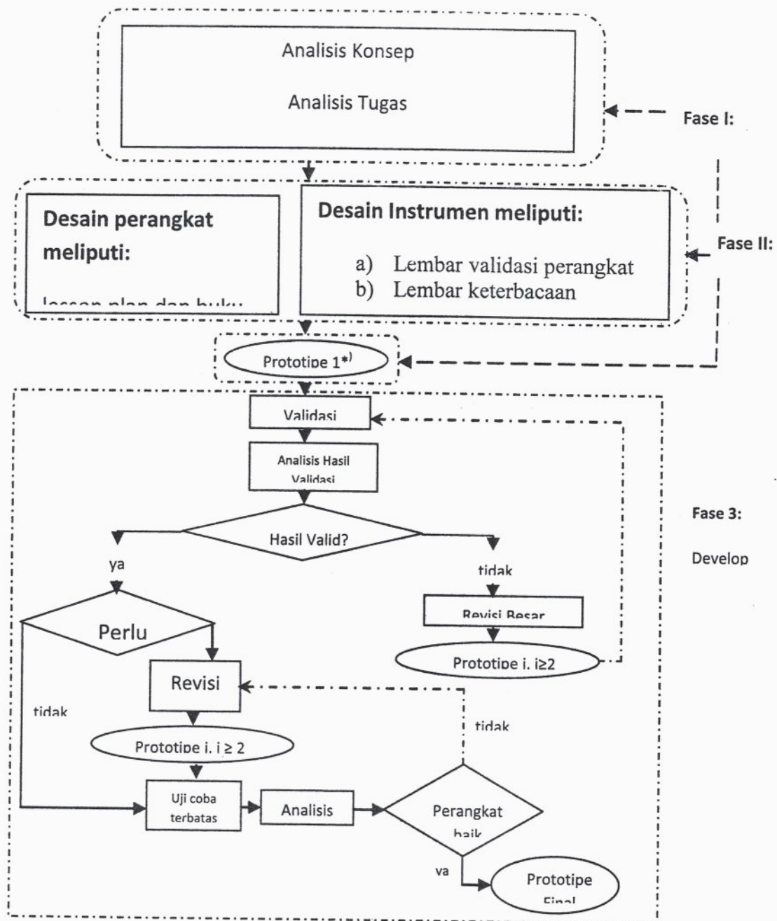
Gambar 1 Diagram ALur Fase Pengembangan
